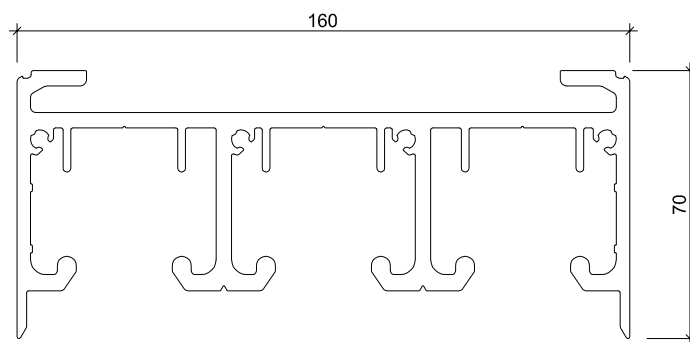
Art. Nr.: 50 9434 Bezeichnung: Oberschiene 3-bahnig Aluminium
