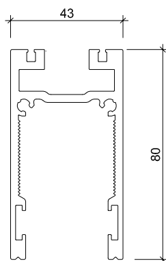
Art. Nr.: 50 9226 Bezeichnung: Laufsuh oben Aluminium
