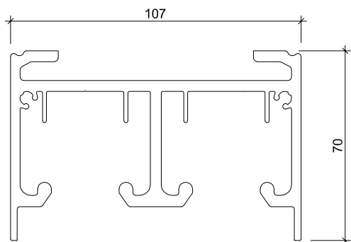
Art. Nr.: 50 9424 Bezeichnung: Oberschiene 2-bahnig Aluminium
