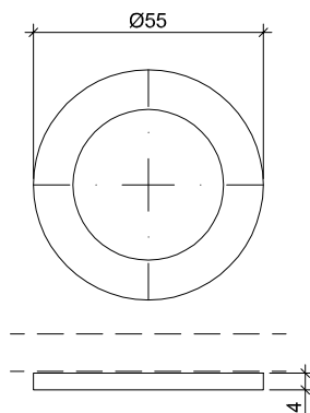
Art. Nr.: 56 6310 Bezeichnung: CNS-Ring Edelstahl UV-verklebt (nur Innenseite)
