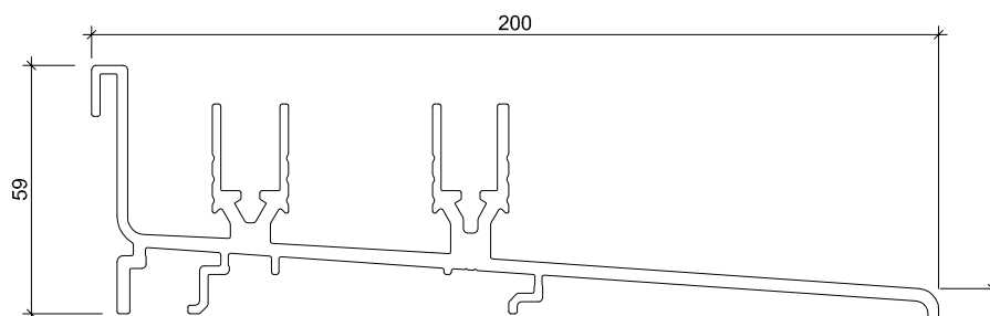
Art. Nr.: 50 9122 Bezeichnung: Wetterbank mit Führung 2-bahnig Aluminium
