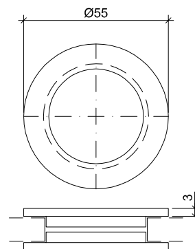
Art. Nr.: 59 0031 Bezeichnung: Muschelgriff beidseitig Edelstahl
