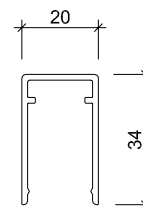
Art. Nr.: 50 9322 Bezeichnung: Klipsprofil Aluminium eloxiert
