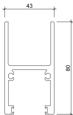
Art. Nr.: 50 9218 Bezeichnung: Laufsuh unten Aluminium
