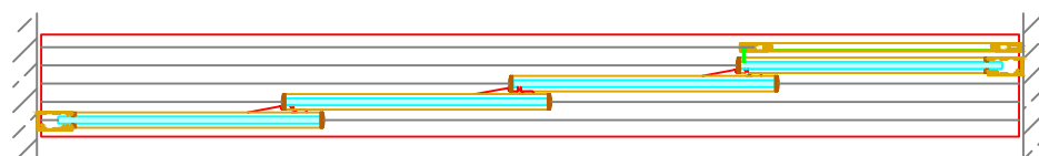
Zustand Glasschiebeelemente geschlossen
