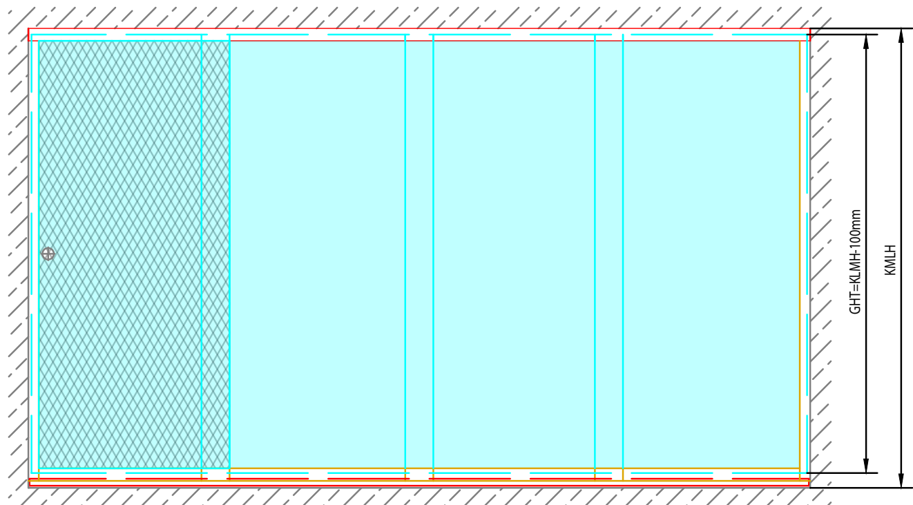
5 Bahnen, 4 Schiebeelemente
