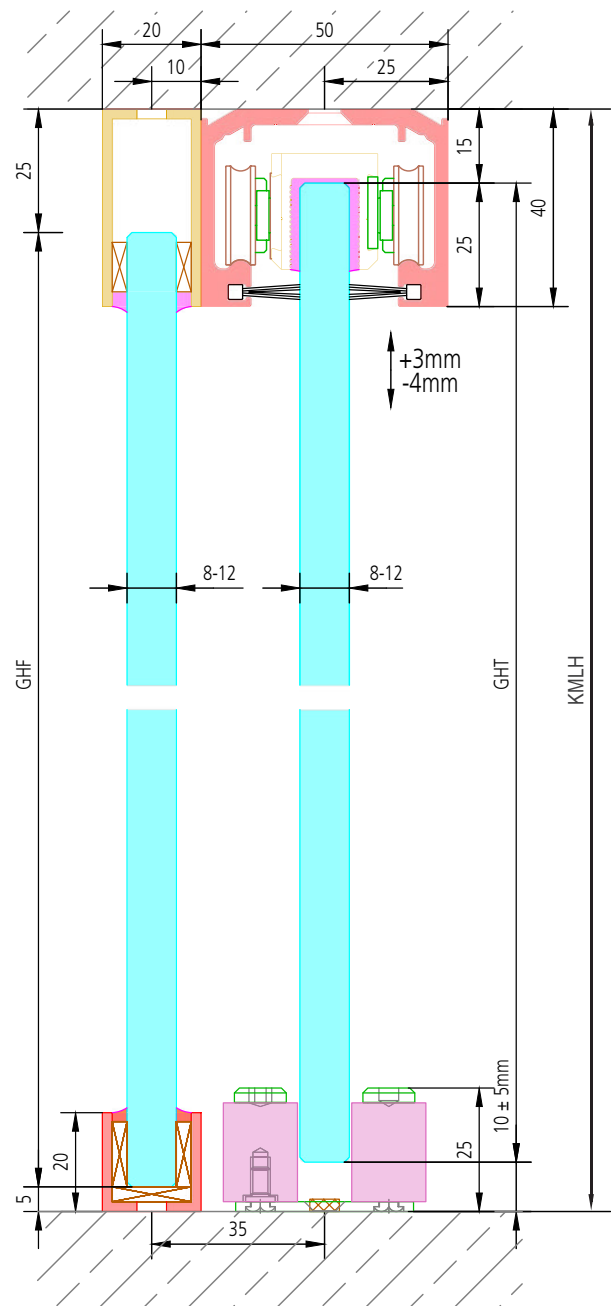
Deckenmontage mit Festverglasung
