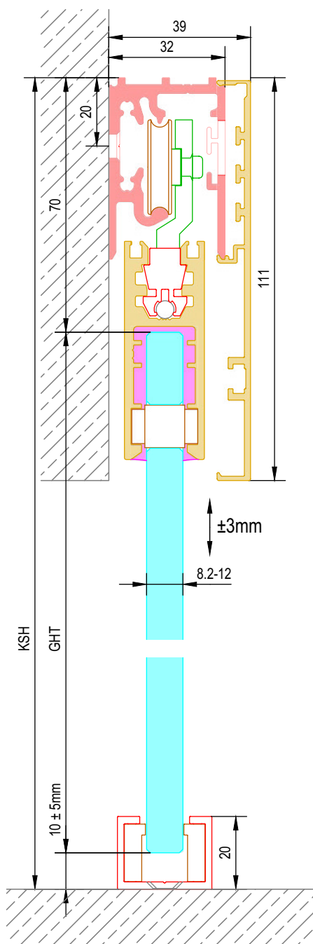
Wandmontage mit Abdeckblende hoch
