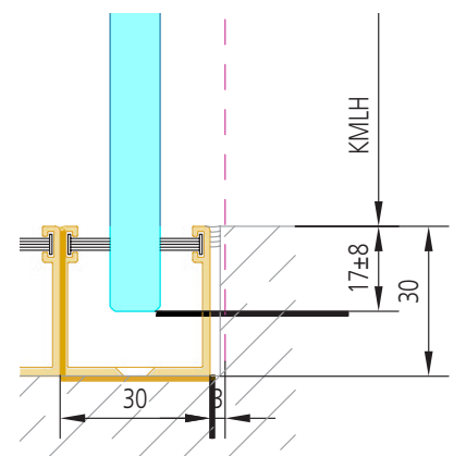
Variante mit Bodenführung (2- bis 4-bahnig)
