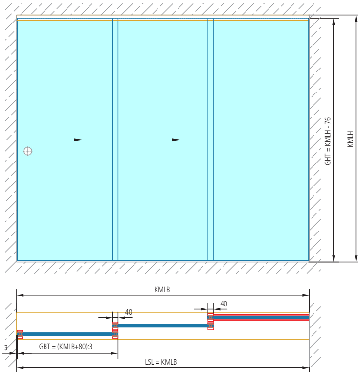
Schiebeanlage zwischen Wand
